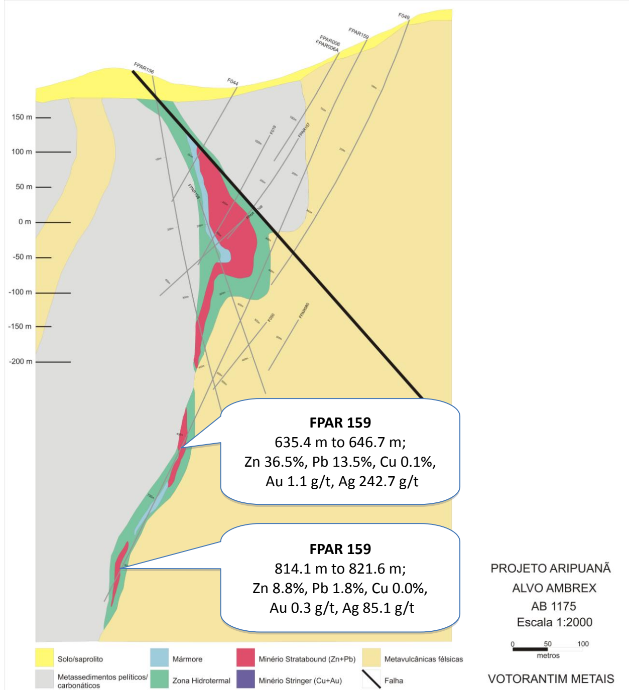
Figura 2; Resultados de Perforación Profunda en Ambrex
