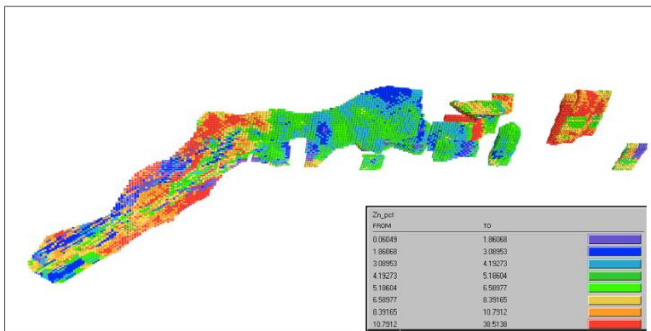
Figura 1; Leyes de Zinc de Arex
